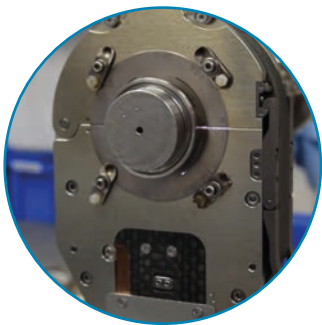
Soudage orbital automatisé dans un environnement à air contrôlé dédié
